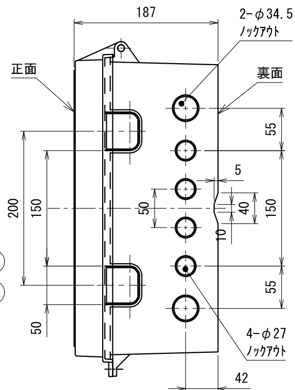
底面図
